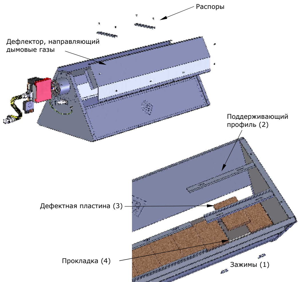
Рисунок 4.5 Замена каталитических пластин
