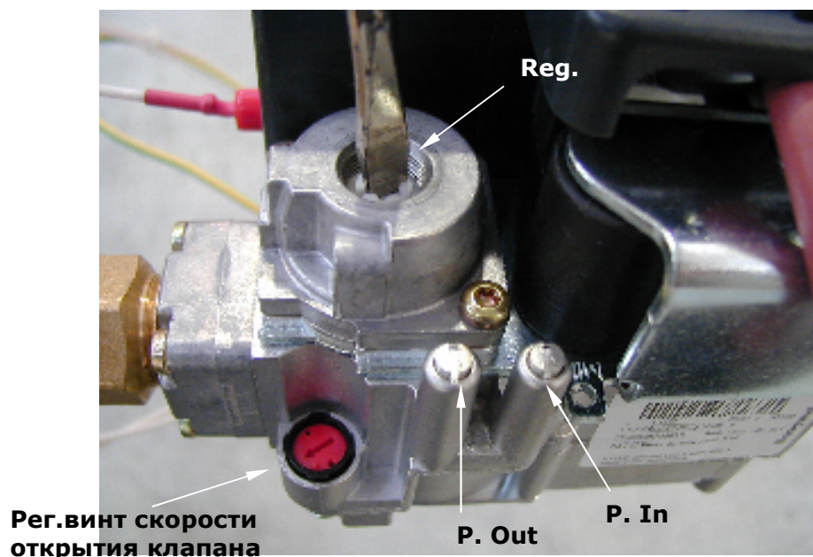
Рисунок 4.1 Установка давления модели с клапаном HONEYWELL
