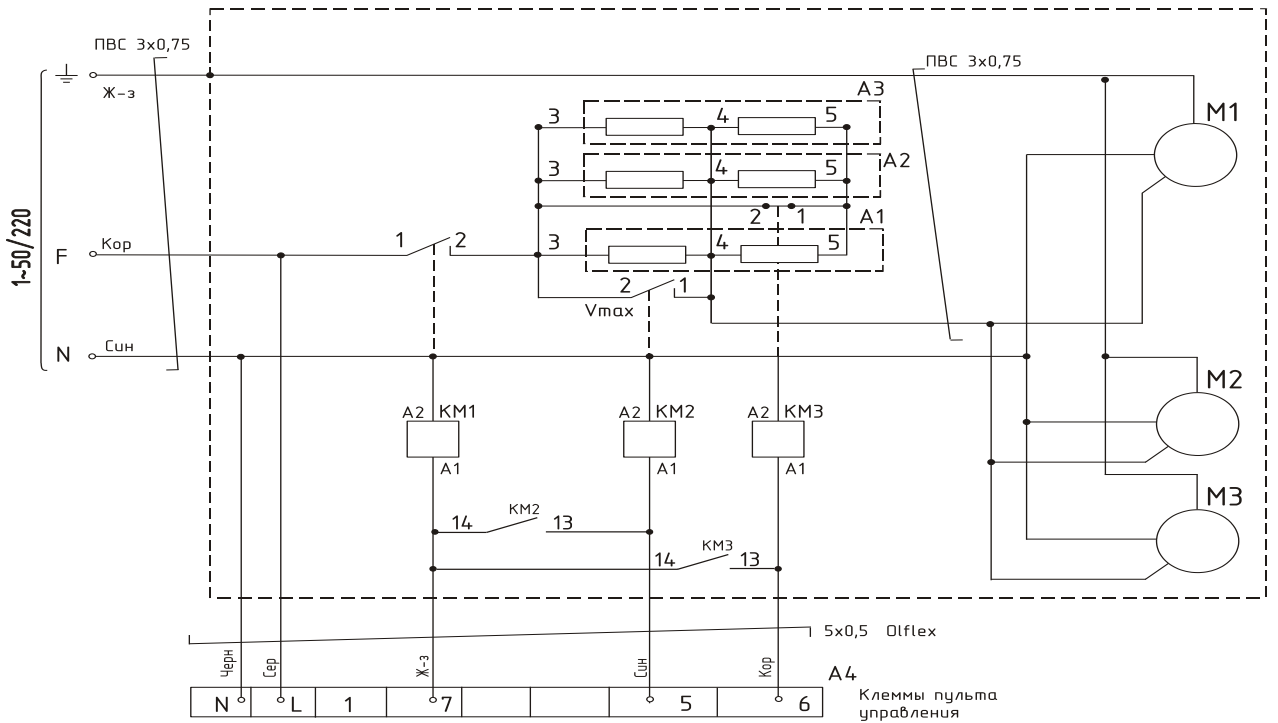
ТЭН-резистор A1..A3
