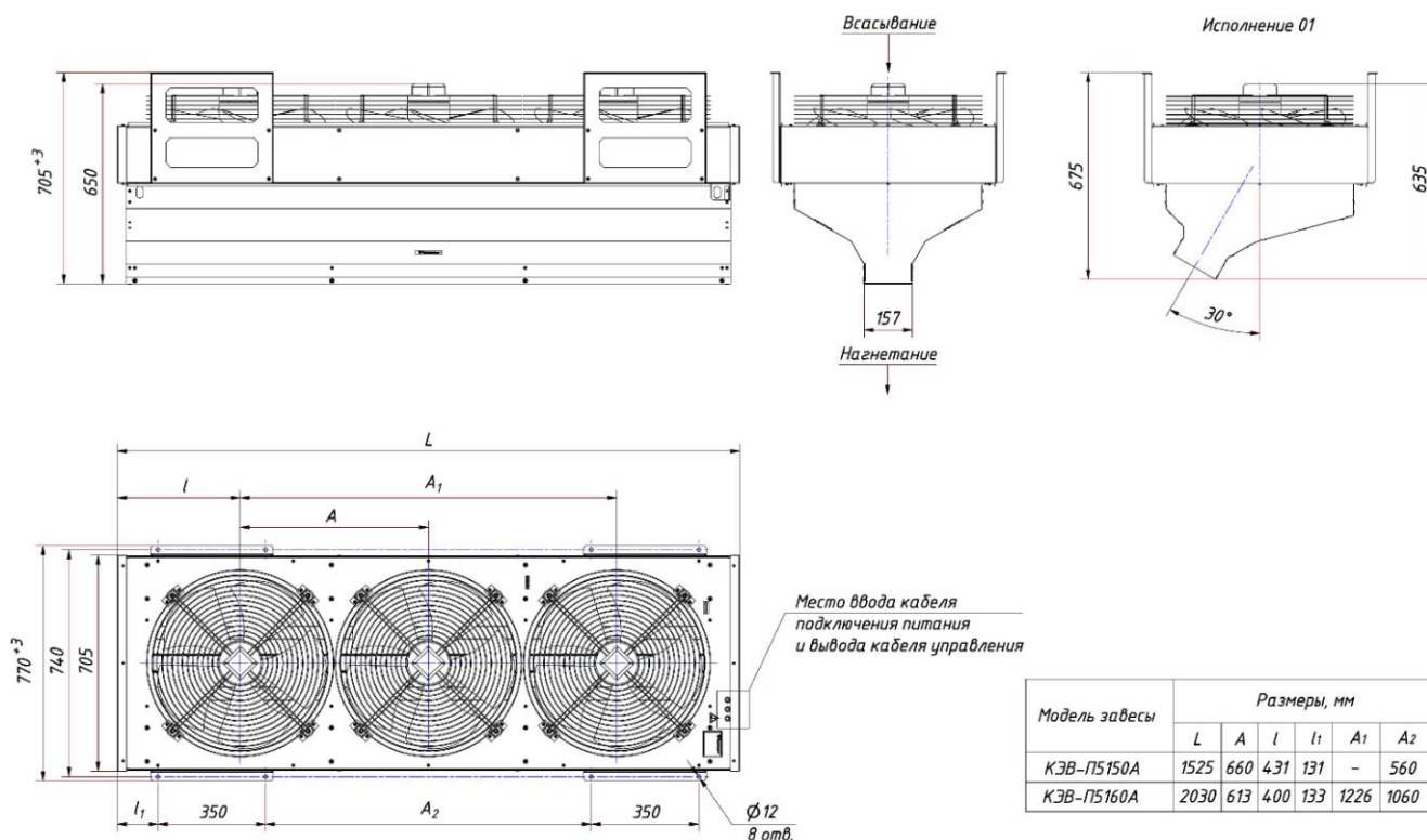
Рис. 8. Крепежные и габаритные размеры КЭВ-П5050А, КЭВ-П5060А
