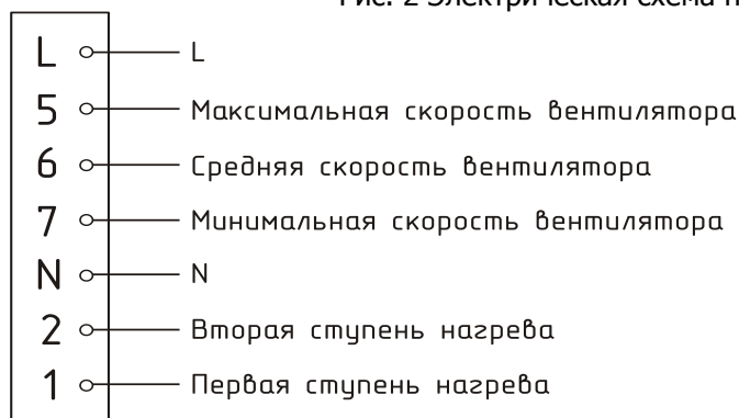
Рис. 2 Электрическая схема подключения пульта управления
